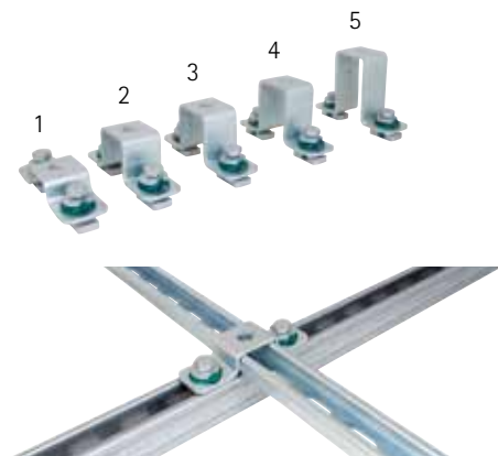
Walraven RapidStrut® Kreuzverbinder G2 (BUP1000)
