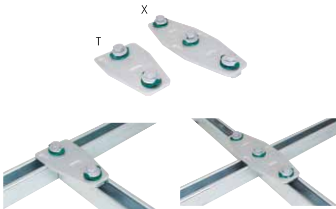
Walraven RapidStrut® Schienenverbinder T und X G2 (BUP1000)
