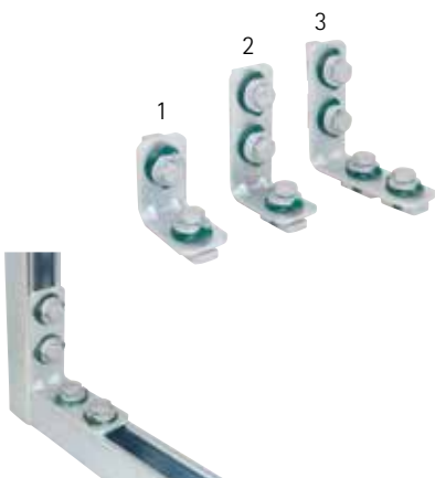
Walraven RapidStrut® Schienenverbinder 90° G2 (BUP1000)
