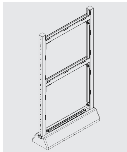
Leitungsführung / Kabelpritschen Ausführung doppelt
